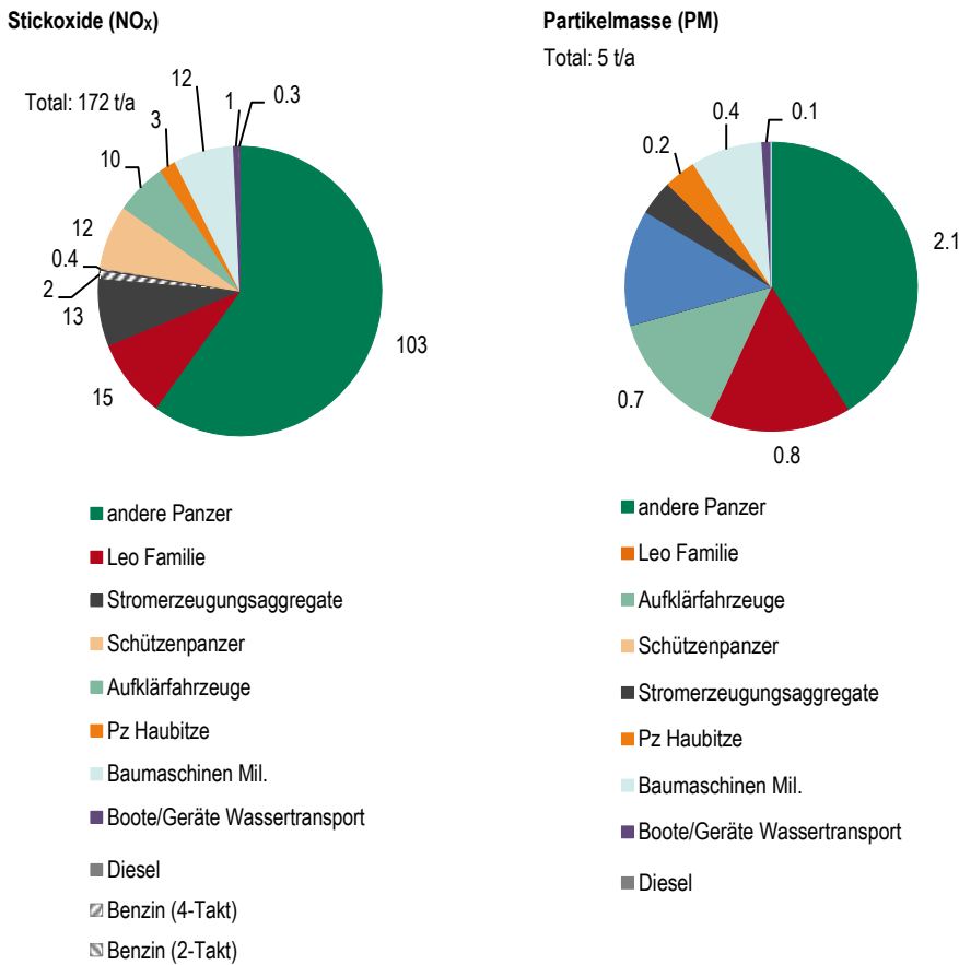
Abb. 55 > Militär: Emissionen im Jahr 2010 und zeitliche Entwicklung (1980–2050)
